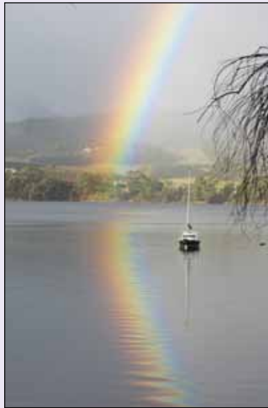
Figuur 8: regenboog en weerspiegeling daarvan in water. Net als in figuur 1 krult de weerspiegeling bij de horizon naar binnen. Foto: Peter Shanks, Hobart, Tasmanië, Australië, 18 juli 2010. (Bron: Flickr)
