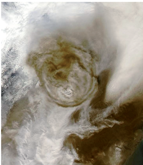
Figuur 2. Satellietbeeld van de uitbarsting van de Grímsvötn op IJsland. Datum 22 mei 2011. Instrument: MODIS satelliet Terra (bron: NASA/University of Dundee).
