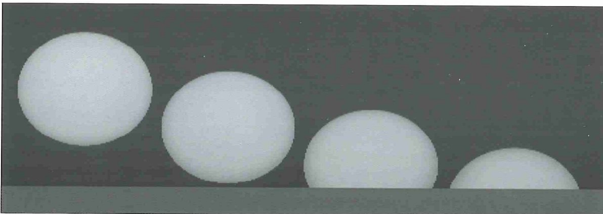
Figuur 1. Computersimulatie van een 'normale' zonsondergang door Dan Bruton (1996). De gehanteerde temperatuuroopbouw van de dampkring is volgens de zogeheten U.S. Standaardatmosfeer. Het beeld dat de atmosfeer vormt van de zonneschijf is afgeplat.
