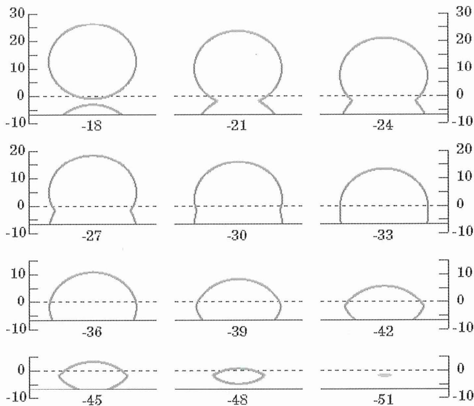
Figuur 2. Computersimulatie van een zonsondergang boven warm zeewater door Andrew Young (1999). De gehanteerde temperatuuropbouw van de dampkring is volgens de U.S. Standaardatmosfeer, met uitzondering van de onderste paar meter, die enkele graden warmer werden genomen. De getrokken horizontale lijn is de kim of de zogeheten optische horizon (Fraser 1975). De streepjeslijn is de astronomische horizon. De getallen onder de berekende vormen van de zonnescijf geven de werkelijke hoogte aan van het middelpunt van de zon in boogminuten; door zogeheten atmosferische straalkromming staat het beeld dat de atmosfeer van de zon vormt, echter hoger aan de hemel. De hoogte waarop we het beeld zien, is af te lezen langs de verticale as; ook hier is de eenheid boogminuten. De hoogte van de astronomische horizon bedraagt 0 boogminuten; negatieve waarden hebben betrekking op posities onder de astronomische horizon. De horizontale diameter van de zon (en bij hoge zonnestanden natuurlijk ook de verticale diameter) bedraagt 32 boogminuten. Bij een zonshoogte van -18 boogminuten (figuur linksboven) is de weerspiegeling zichtbaar van het onderste gedeelte van de zonnescijf in de warme laag direct aan het aardoppervlak. Bij zonshoogten van -21 boogminuten of lager vormen de zonnescijf en zijn weerspiegeling een geheel. Eerst ontstaat de karakteristieke vorm van de Griekse hoofdletter omega [zonshoogten van -21 en -24 boogminuten]; later lijkt het of er deuken zitten in het onderste deel van de zonnescijf [-27, -30]. Als de zon zich 33 boogminuten onder de horizon bevindt, zijn de deuken verdwenen en lijkt het beeld van de zonnescijf in verticale richting uitgerekt; daarna vertoont het laatste segment dat van de zon zichtbaar is, afgeronde hoeken. Uiteindelijk verdwijnt de zon bij een zonshoogte van ruim 51 boogminuten, echter niet aan de kim, maar iets daarboven.
