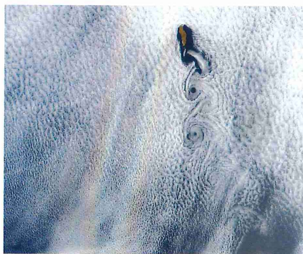
Figuur 10. Satellietbeeld van een langgerekte glorie 'rond' het met de satelliet mee bewegende tegenpunt van de zon. Het lichteffect is zichtbaar in stratocumulusbewolking boven de Grote Oceaan voor de kust van Baja California, Mexico. Achter het eiland Guadalupe zijn Von Kármánwervels zichtbaar. Datum: 20 juni 2012, instrument: MODIS, satelliet: Aqua (bron: NASA).
